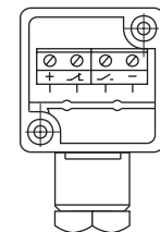
Маркировка клемм
